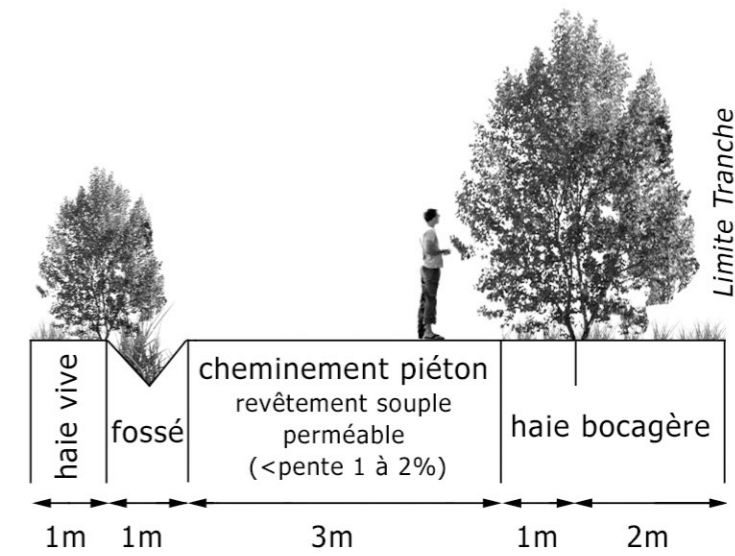
Coupe C7 (emprise : 8 m)
