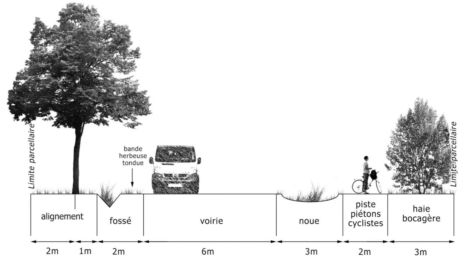
Coupe C3 (emprise : 19 m)
