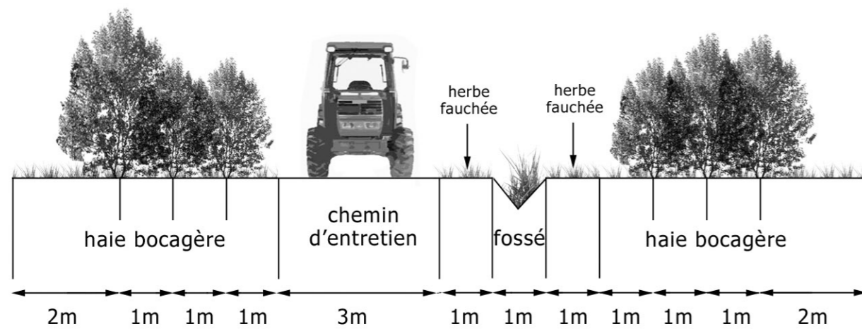
Coupe C8 (emprise : 16 m minimum)
